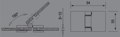
REFERÊNCIA: DB11B ESCOVADO/POLIDO DOBRADIÇA VIDRO/VIDRO COM ABERTURA NOS DOIS SENTIDOS
