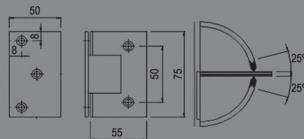
REFERÊNCIA: DB4B MATE/BRILHO DOBRADIÇA VIDRO/PAREDE COM ABERTURA NOS DOIS SENTIDOS
