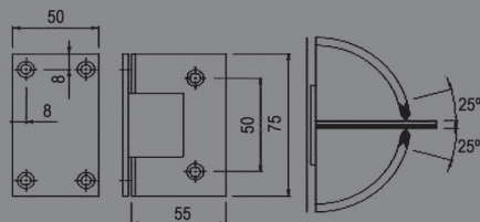
REFERÊNCIA: DB4A MATE/BRILHO DOBRADIÇA VIDRO/PAREDE COM ABERTURA NOS DOIS SENTIDOS
