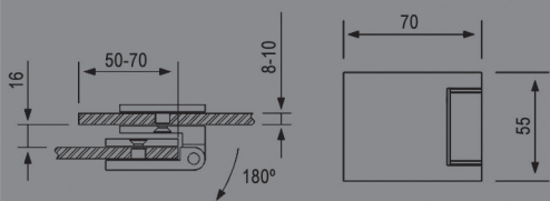
REFERÊNCIA: DB11C ESCOVADO/POLIDO DOBRADIÇA VIDRO/VIDRO COM 1 SENTIDO DE ABERTURA
