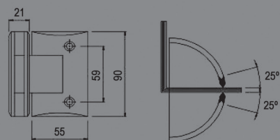
REFERÊNCIA: DB3D MATE/BRILHO DOBRADIÇA VIDRO/VIDRO 90° COM ABERTURA NOS DOIS SENTIDOS
