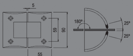
REFERÊNCIA: DB3C MATE/BRILHO DOBRADIÇA VIDRO/VIDRO COM ABERTURA NOS DOIS SENTIDOS
