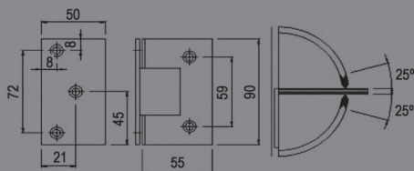
REFERÊNCIA: DB3B MATE/BRILHO DOBRADIÇA VIDRO/PAREDE COM ABERTURA NOS DOIS SENTIDOS
