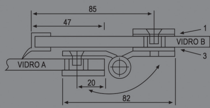
REFERÊNCIA: DB9B ESCOVADO/POLIDO DOBRADIÇA VIDRO/VIDRO COM 1 SENTIDO DE ABERTURA
