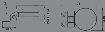
REFERÊNCIA: DB8A BRILHO DOBRADIÇA VIDRO/PAREDE COM 1 SENTIDO DE ABERTURA
